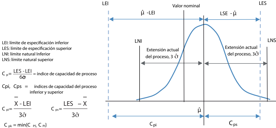
Figura 6.3. Modelo de análisis gráfico de la capacidad del proceso
