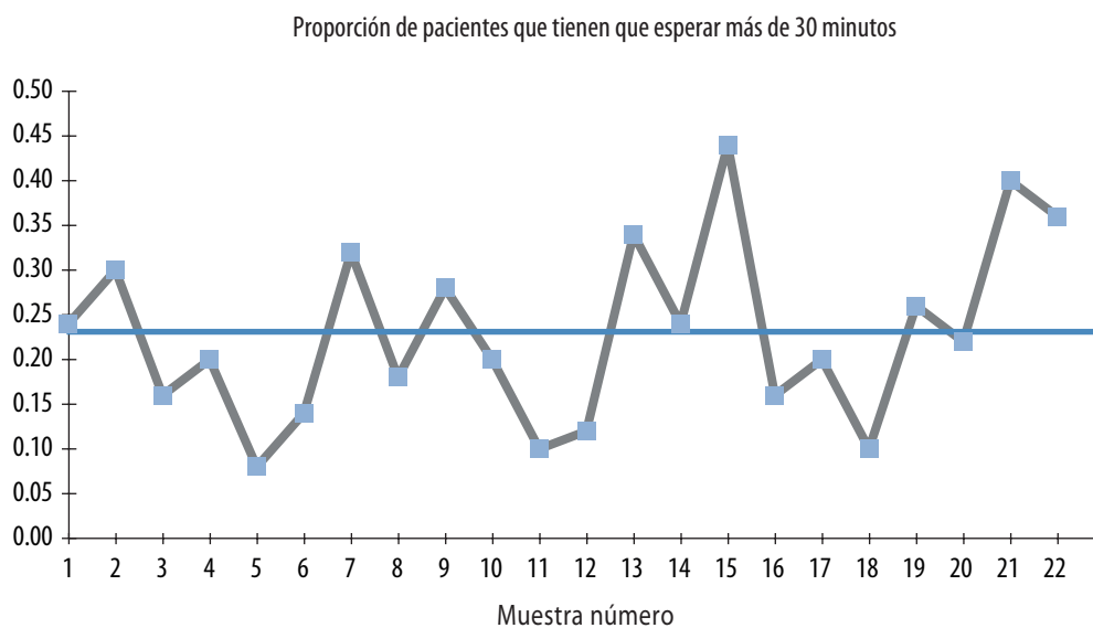
Figura 4.5. Gráfico de rachas ( run chart ) para el indicador "proporción de pacientes que tienen que esperar más de 30 minutos" 1x
